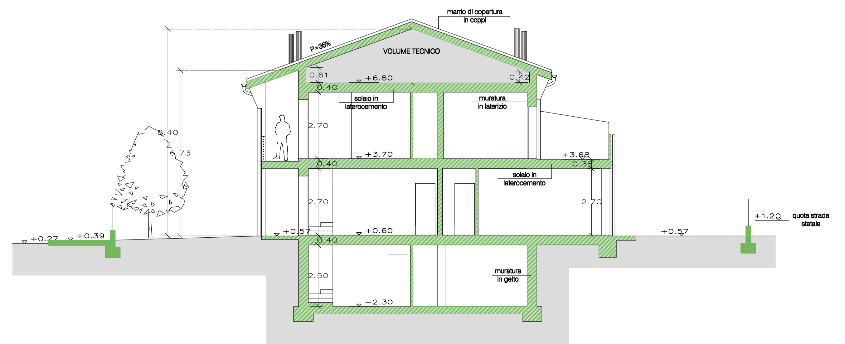
SEZIONE B-B
