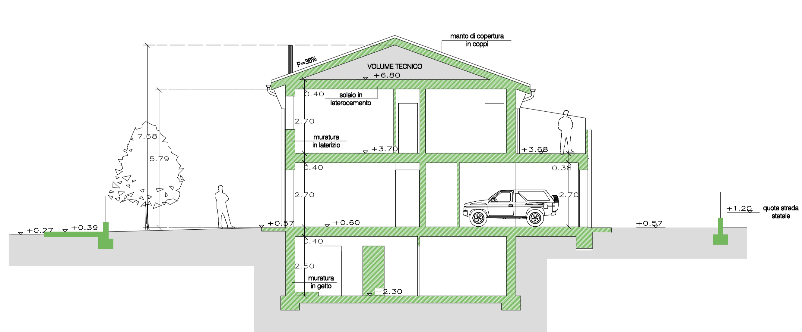
SEZIONE A-A
